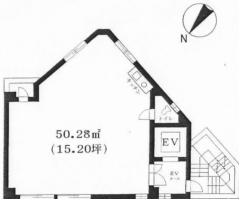
【2階平面図】
